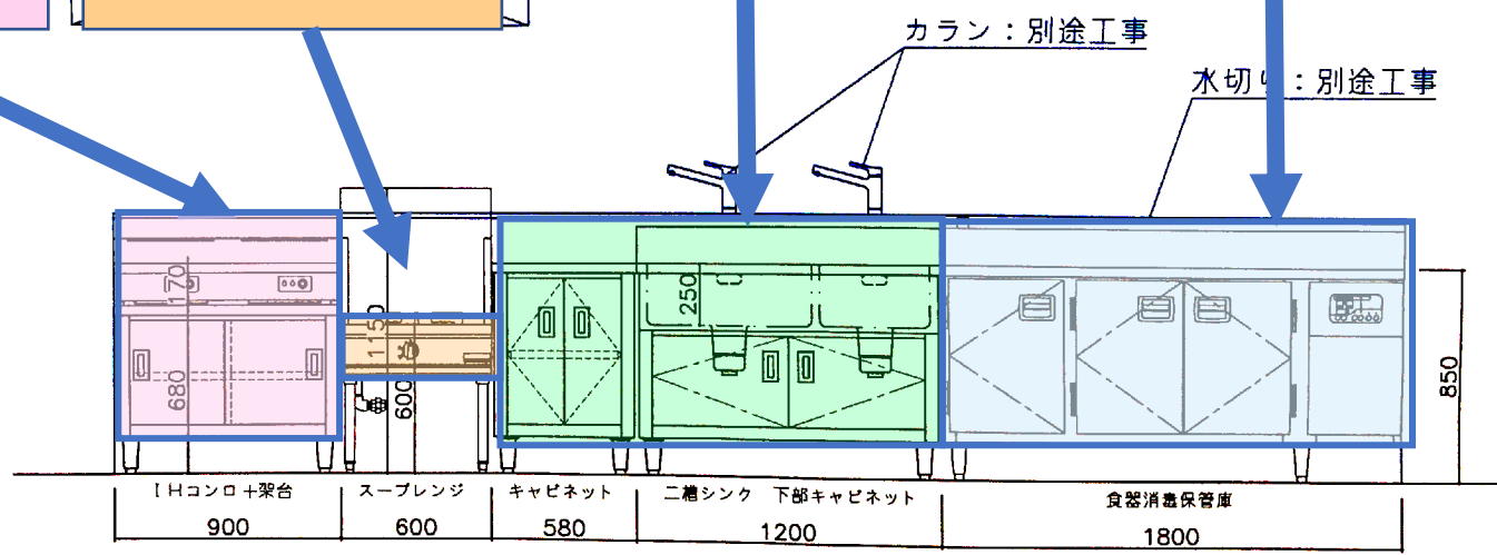
展開図
