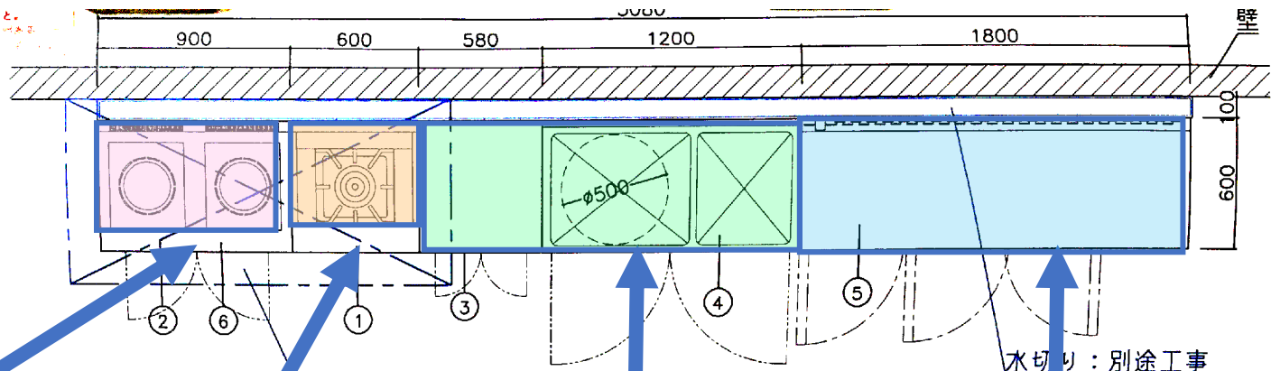
平面図
